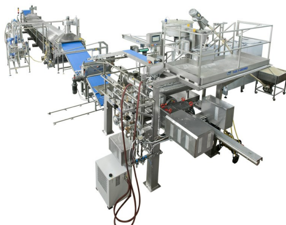
■ Модуль варки со штоками на линии предварительной варки листов b
